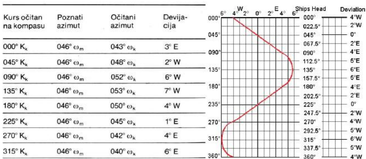
Tablica i krivulja devijacija magnetskog kompasa na brodici
