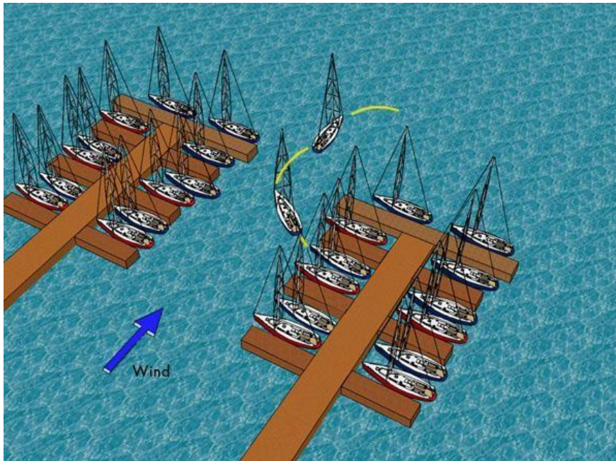
Manevar isplovljenja
